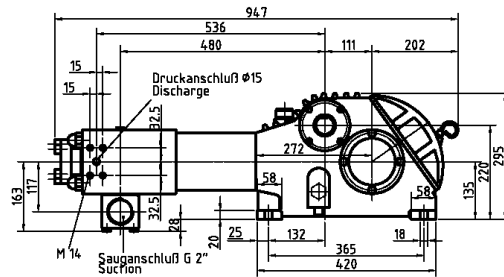
Hochdruckkopf A High Pressure Head A
